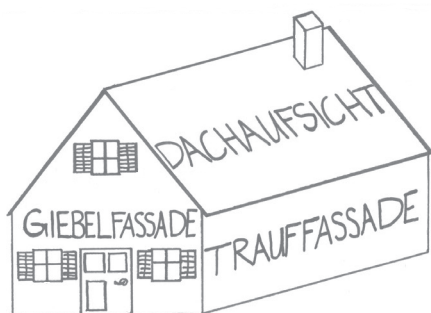
Abbildung 3: Hausansichten
